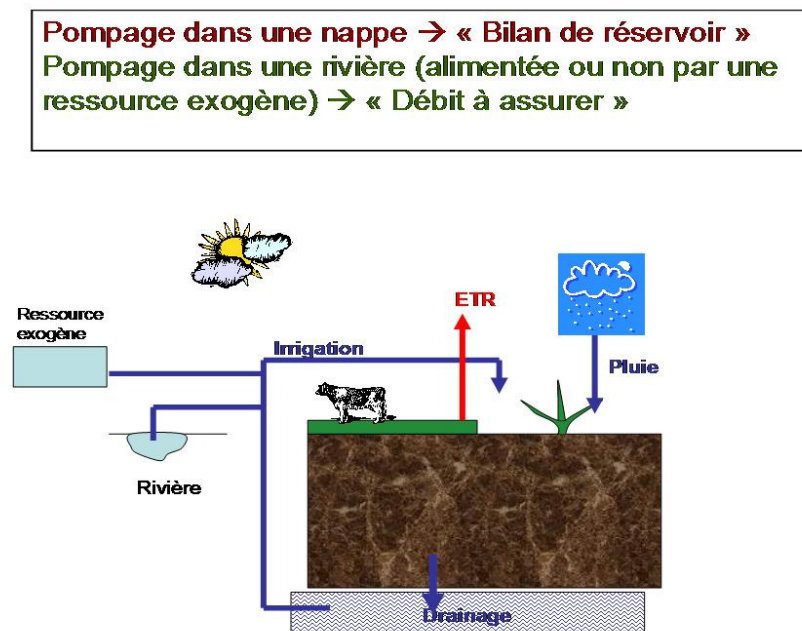
Figure 2 : Deux situations très contrastées : pompage dans une nappe et pompage dans une rivière
